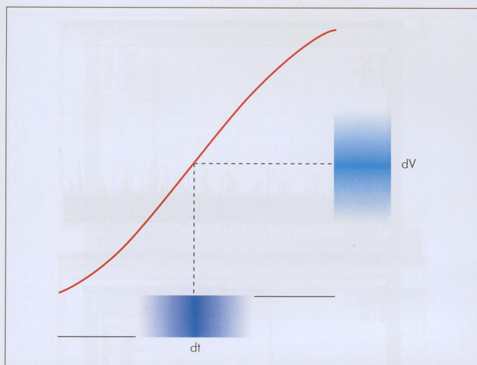
Рис.1. Влияние нестабильности частоты тактового сигнала на точность измерения амплитуды
