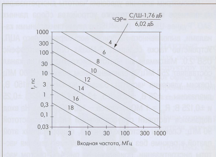
Рис.2. Влияние джиттера на число эффективных разрядов в зависимости от частоты входного сигнала
