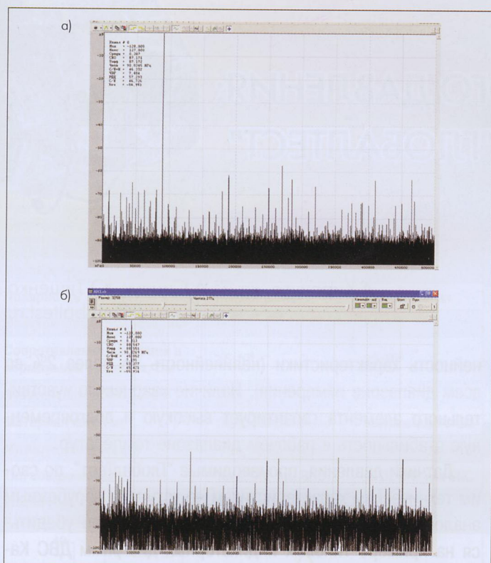
Рис.5. Спектральные характеристики платы ЛА-н1USB в режиме без удвоения частоты (а) и режиме удвоения частоты дискретизации (б)
