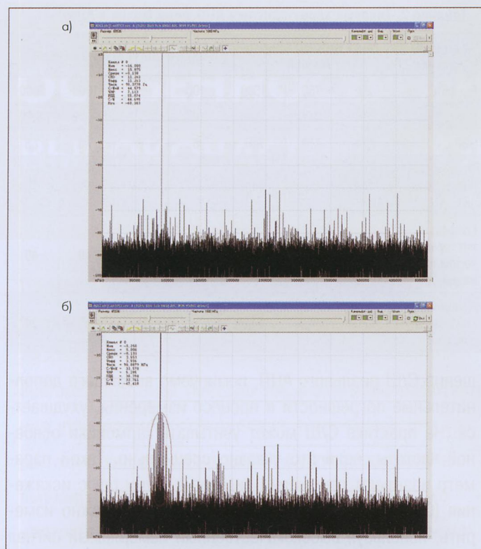
Рис.3. Результаты БПФ при использовании в качестве источника тактовой частоты платы ЛА-н1РС1 стабильного кварцевого генератора (а) и генератор с высоким фазовым шумом (б)
