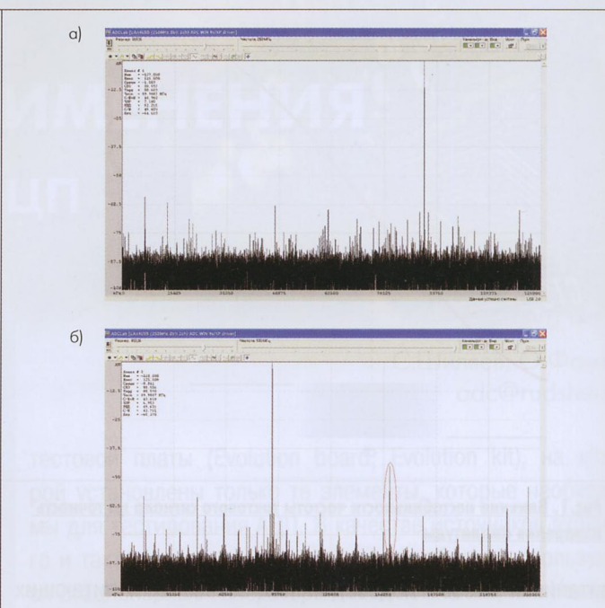
Рис.4. Спектры сигналов, оцифрованных платой ЛА-н4USB в режимах без удвоения (а) и удвоения частоты дискретизации (б). Красной огибающей отмечена спектральная составляющая, появляющаяся из-за различия каналов АЦП
