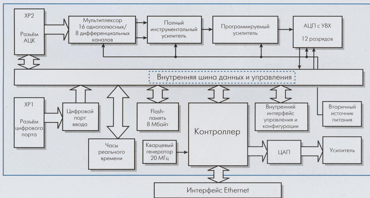
Рис.1. Структурная схема ЛА-5
