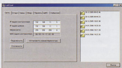
Рис.4. Интерфейс программы La5Conf (вкладка "Сеть")
