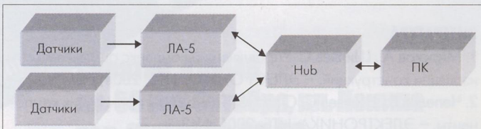
Рис.2. Схема измерительно-вычислительной сети с использованием ЛА-5
